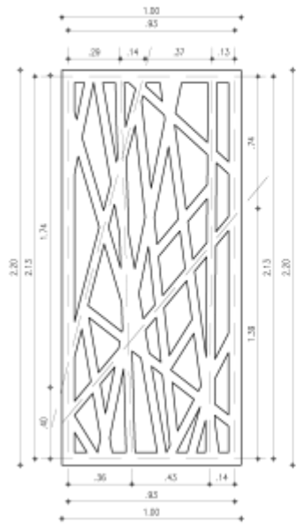
ALZADO
